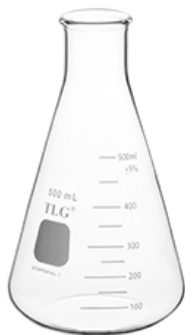
Erlenmeyer Flask
